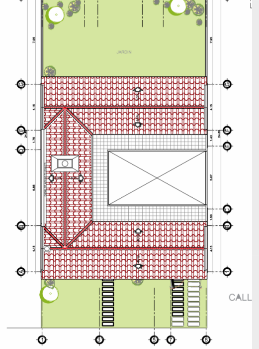
1 Planta - De Cubiertas Cortijo, Lote 19 ESCALA 1:100
